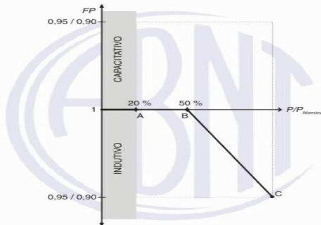
produção Graph potência reativa de acordo com uma curva de Fator de Potência característica Graph reactive power production according to a characteristic Power Factor Curve
